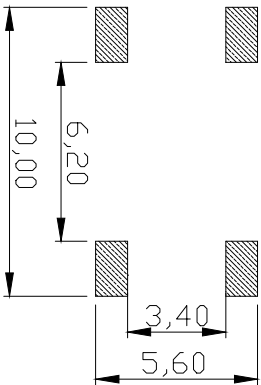
PCB 焊接图
