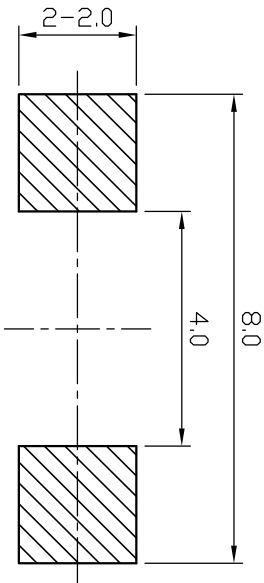
P.C.B. LAYOUT
