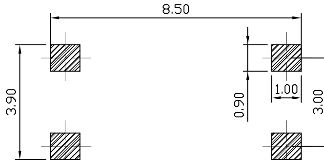
P.C.B LAYOUT
