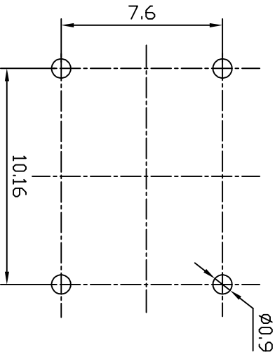
P.C.B. LAYOUT
