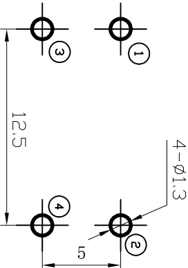
P.C.B LAYOUT
